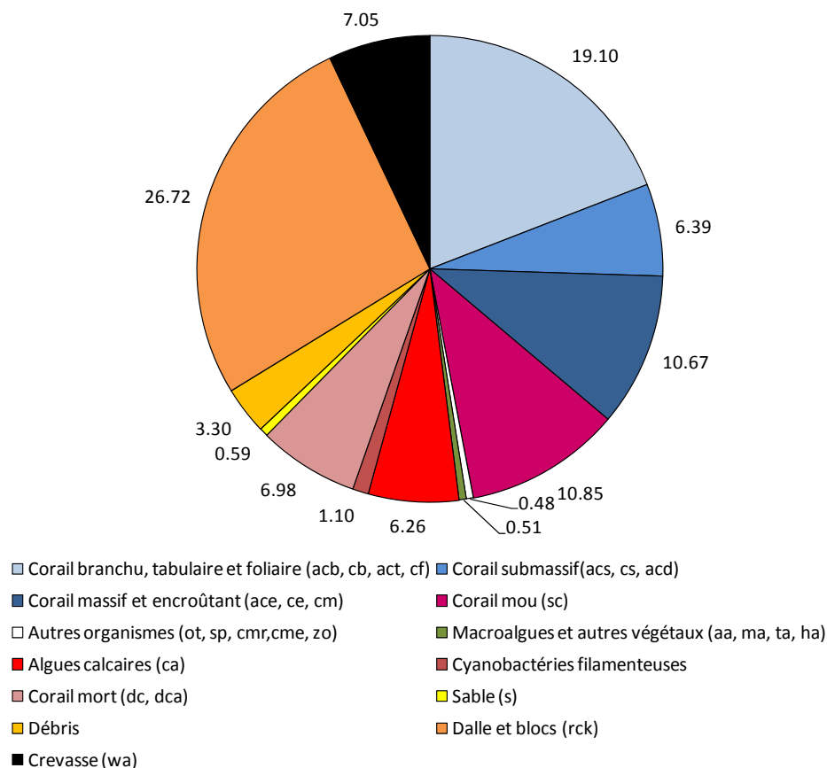
Figure 6 : Caractéristiques moyennes de l'habitat des 8 stations de pente externe dans l'AMP de Yambé/Diaouhé.
