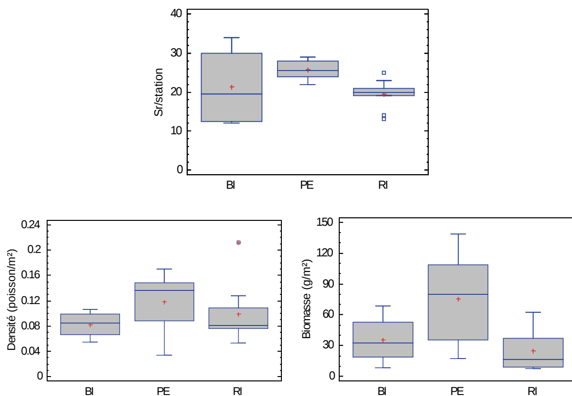
Figure 10: Richesse spécifique par station, densité et biomasse des espèces de poissons commerciaux sur les différents types géomorphologiques de récifs échantillonnés dans l'AMP de Yambé/Diahoué.
