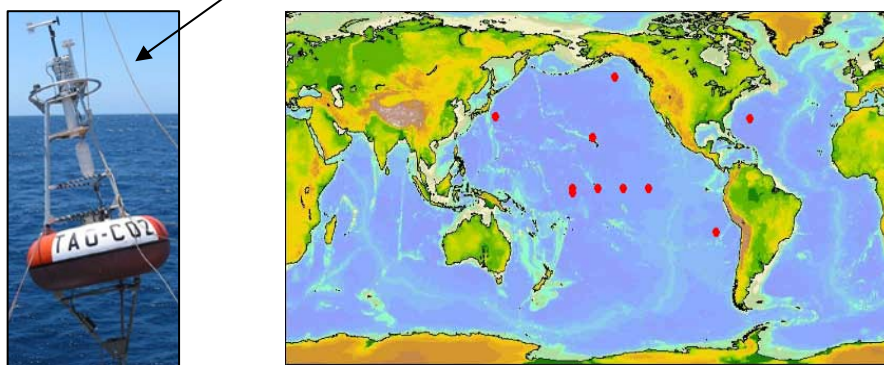
Figure 11 Répartition des bouées TAO dans l'océan mondial
