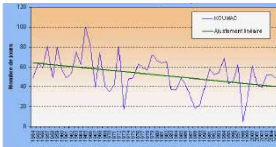
Figure 18. Nombre de jours où la température minimale à été <16°C, à Koumac, sur la période 1951-2005 (tiré de Météo France, 2006 ; 2007).
