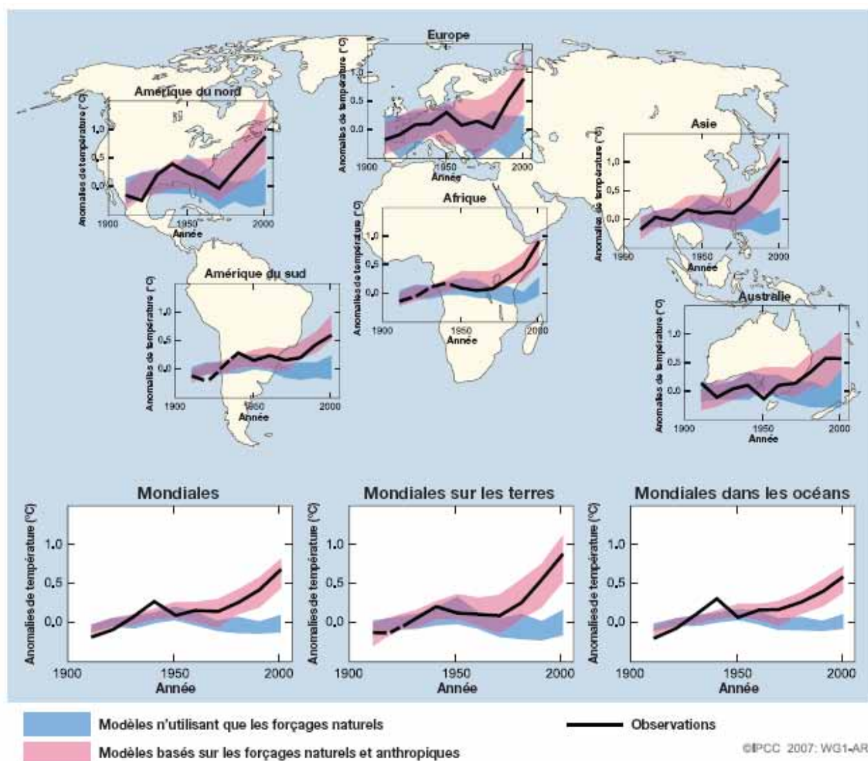
Figure 6. Comparaison des changements observés sur la température de surface aux échelles globale et continentale, avec les résultats de simulations de modèles climatiques utilisant les forçages naturels et anthropiques. Les moyennes décennales des observations sont montrées pour la période 1906–2005 (ligne noire) représentée selon le centre de la décennie et relative à la moyenne correspondante sur la période 1901–1950. Les lignes en pointillés sont utilisées quand la couverture spatiale est inférieure à 50 %. Les bandes bleues ombrées représentent l'intervalle de confiance 5–95% pour 19 simulations de cinq modèles climatiques qui n'utilisaient que les forçages naturels dus à l'activité solaire et aux volcans. Les bandes rouges ombrées représentent l'intervalle de confiance 5–95% pour 58 simulations provenant de 14 modèles climatiques utilisant des forçages à la fois les forçages naturels et anthropiques. (Source : IPCC, 2007)
