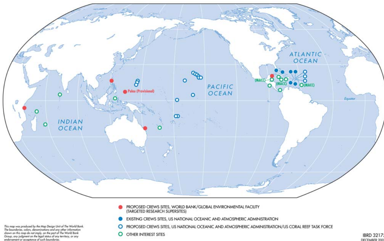
Figure 13. Répartition des stations CREWS existantes ou proposées
