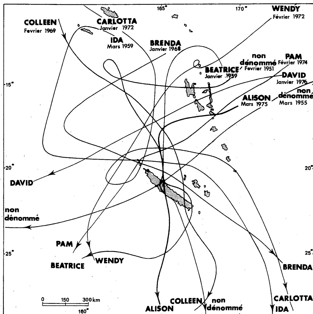
Fig. 2 Trajectoires des cyclones tropicaux ayant intéressé la Nouvelle-Calédonie entre 1951 et 1976
