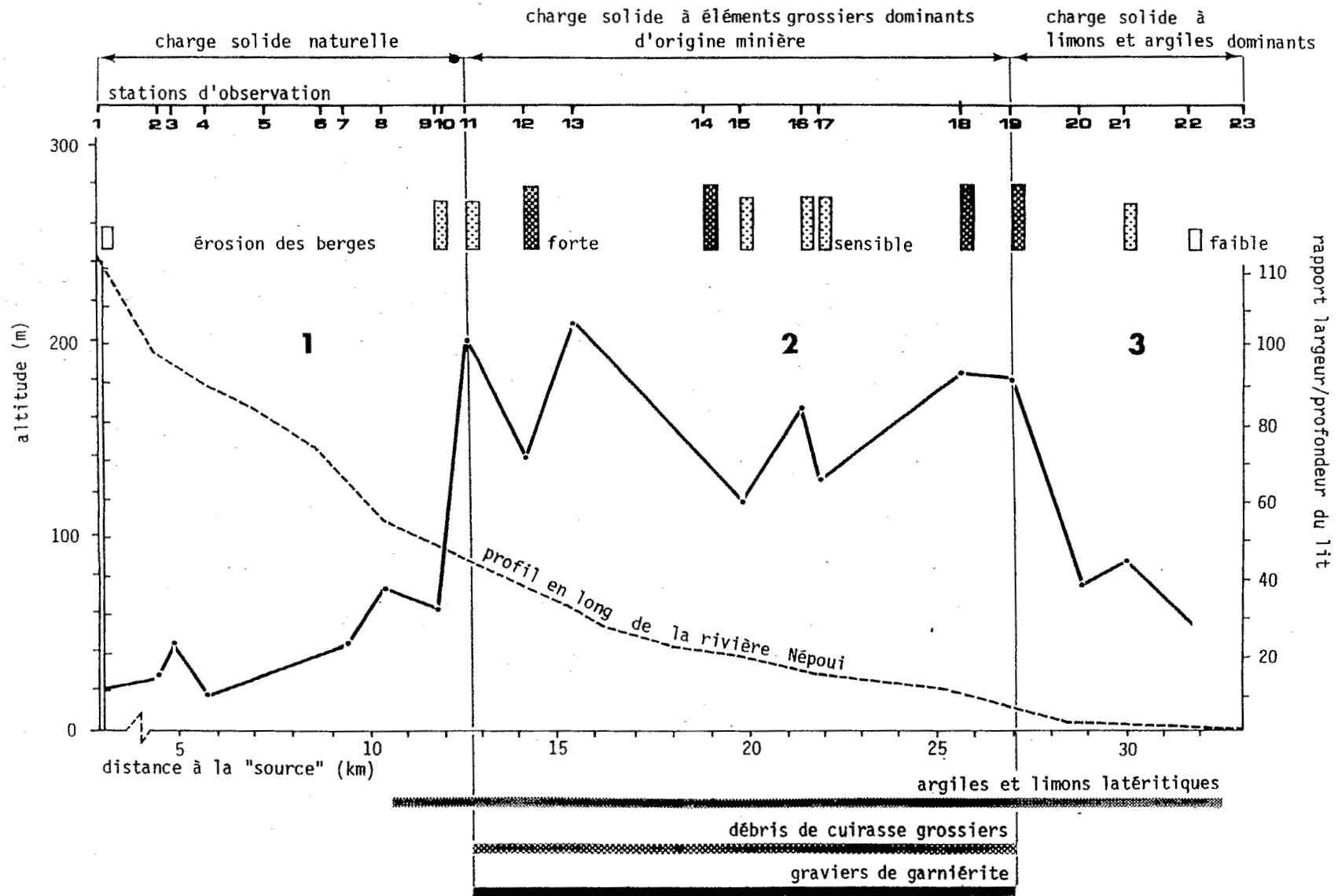
Fig.3 Variation longitudinale du rapport largeur/profondeur du lit actif de la Népoui
