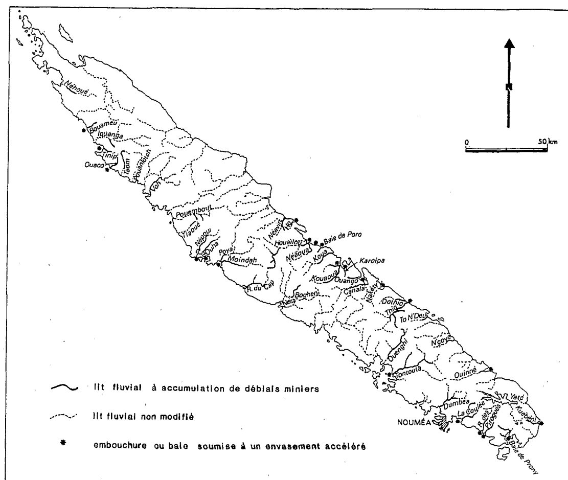
Fig. 4 L'impact des déblais miniers sur le réseau hydrographique et le littoral de la Grande Terre
