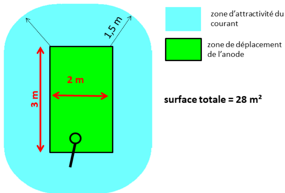
Figure 6 Représentation schématique de la surface prospectée (mouvement de l'anode) et de la surface échantillonnée (efficacité électrique)
