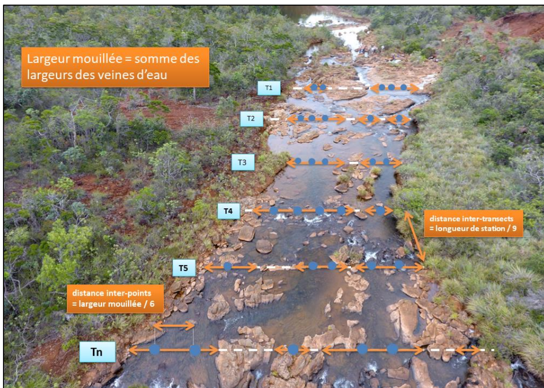
Figure 21 Exemple de réalisation de transects sur une station - en haut sur la Tiwaka (photo J. Bouchard / AFB ), en bas sur le Creek Baie Nord (photo BioEko )
