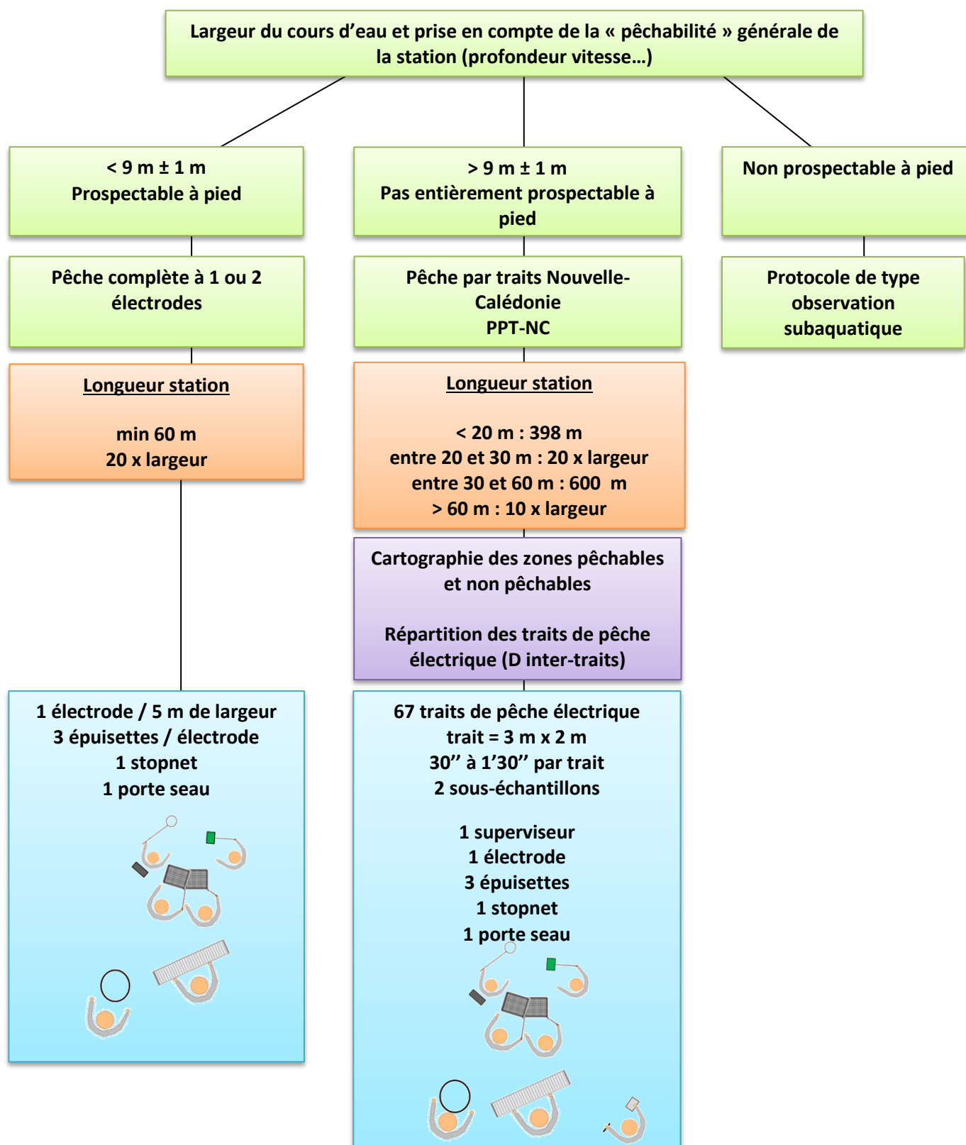
Figure 16 Arbre de décision de la méthode de pêche à mettre en œuvre et des grands principes à respecter en fonction des critères de pêchabilité (largeur, profondeur et vitesses de courant) de la station
