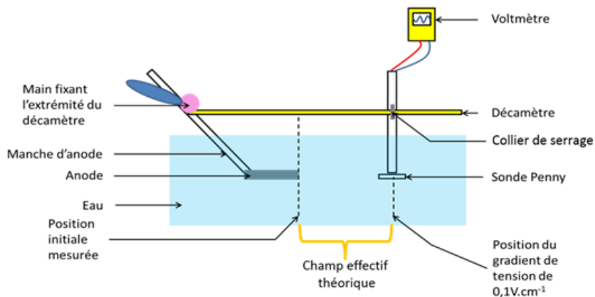
Figure 22 Dispositif de mesure du gradient de tension appelé « sonde penny ». La différence de potentiel est mesurée entre deux électrodes séparées de 10 cm (photo A. Bertaud-OEIL ; schémas extraits de Pottier et al. , à paraître)- Cf. Annexe 3.
