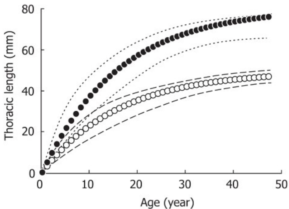
Figure 10 : relation entre taille et âge, à partir de 37 mesures, ajustées par la méthode de Von Bertalanffy (d'après Sato, 2013)
