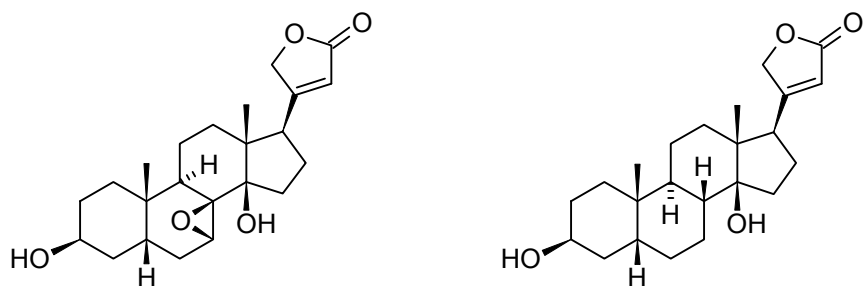
Figures 25 quint & 25 sext : structures de la tanghinigénine et de la cerbérigénine
