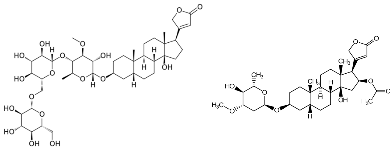
Figure 28 & 28 bis : structures de la thévétine B et de l'oléandrine
