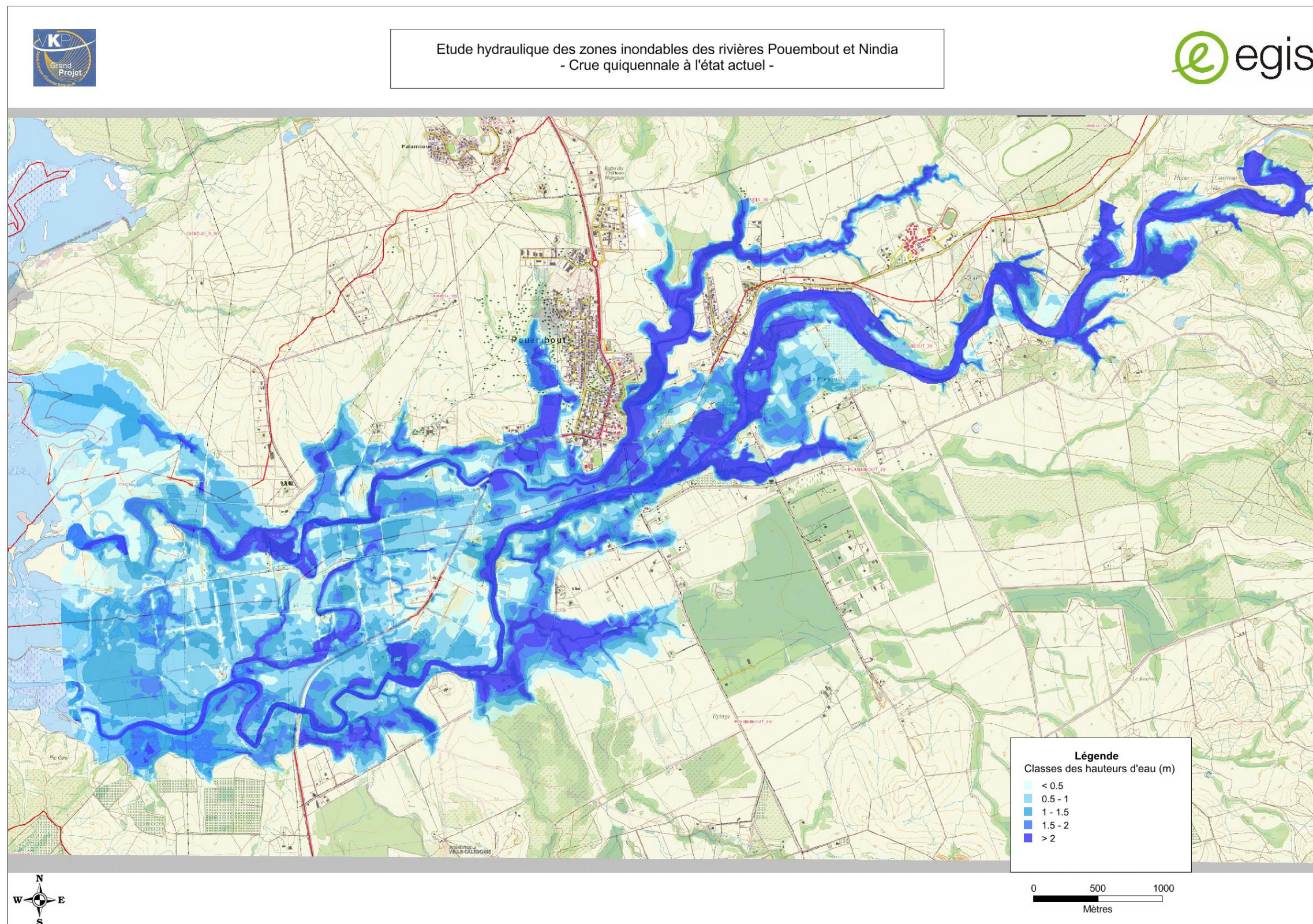
Figure 30 : Cartographie des zones inondables avec iso-hauteurs pour la crue d'ordre de retour Q10 / SactQ10-1
