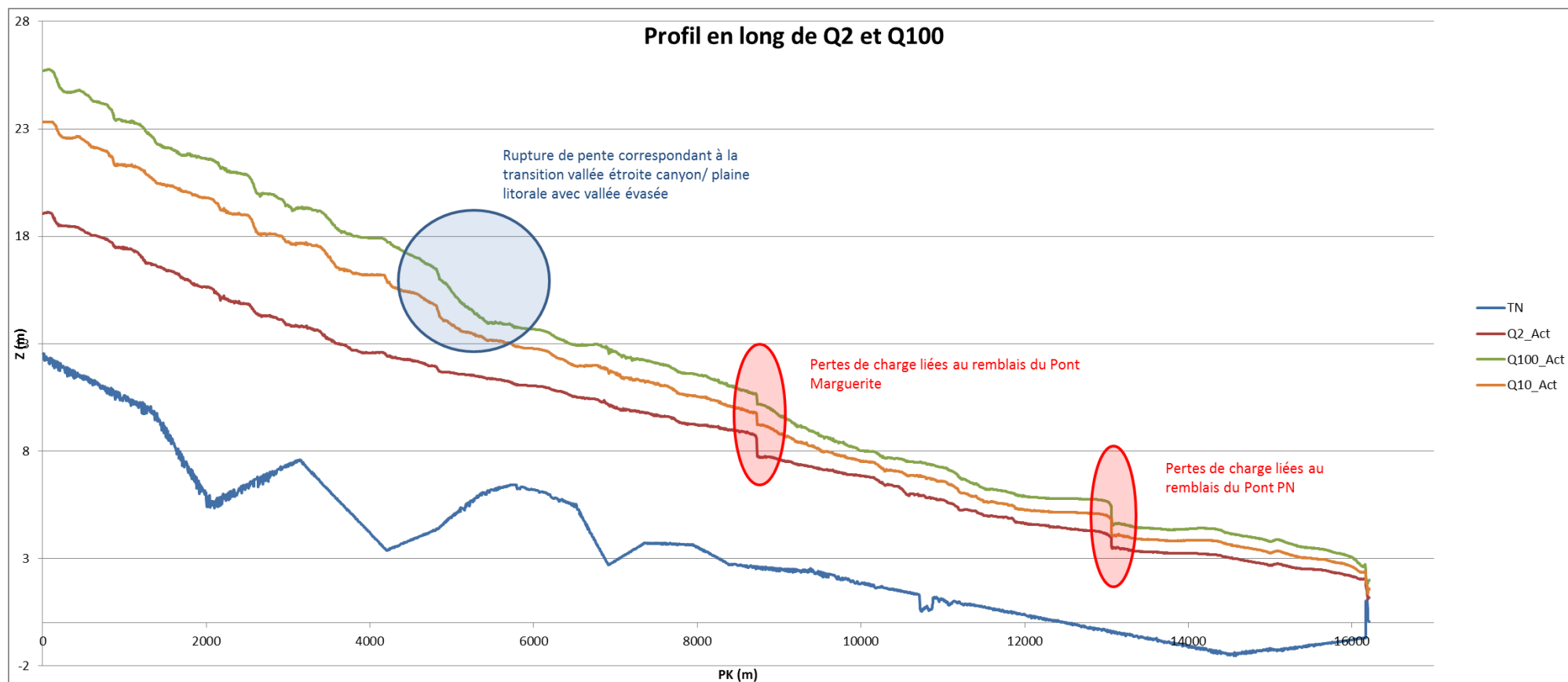
Figure 33 : Profil en long du lit mineur de la Pouembout pour Qi2 et Qi100
