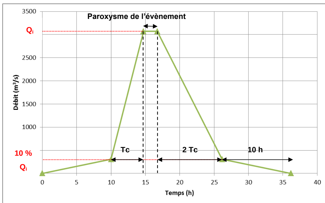
Figure 16 : Description schématique des hydrogrammes reconstitués:
