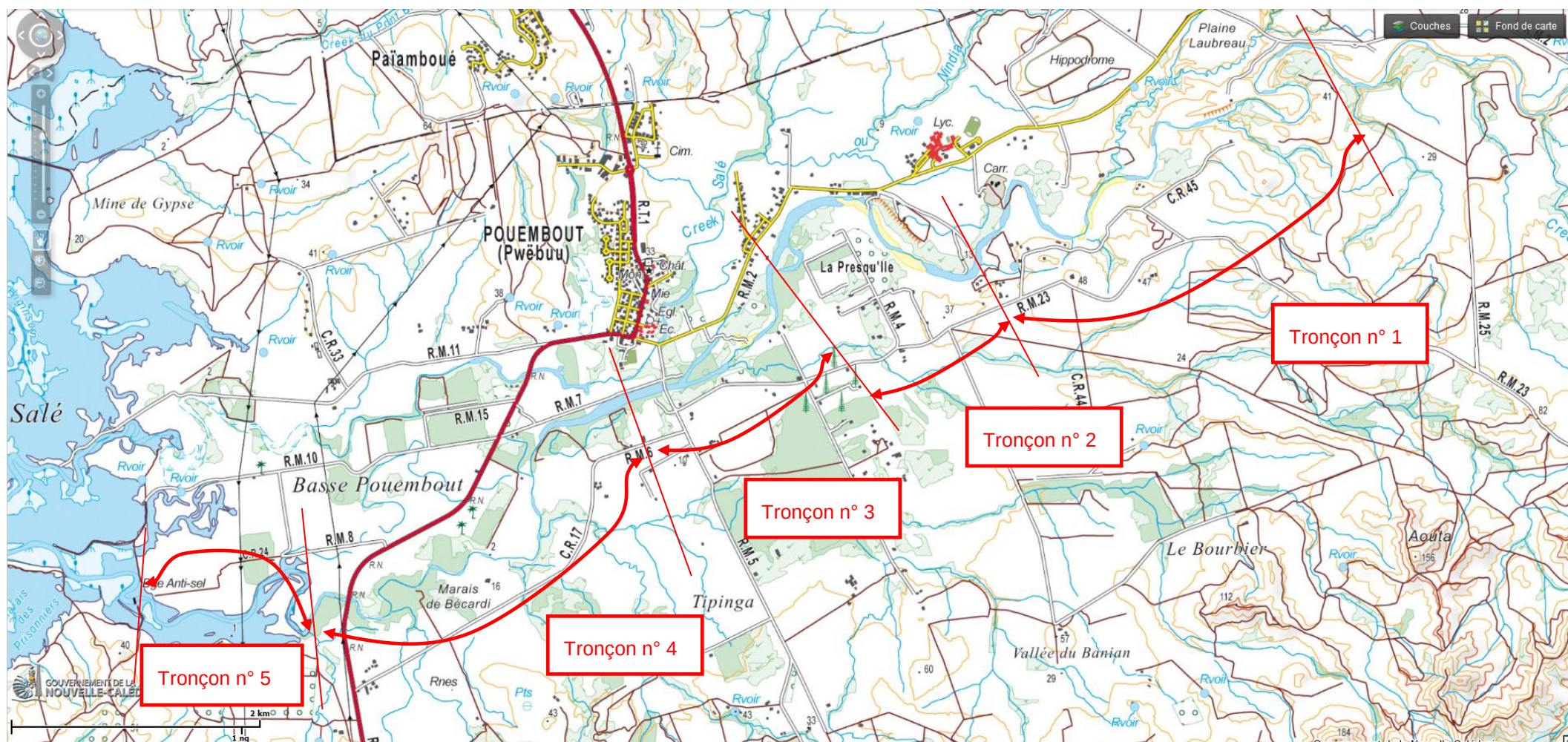
Figure 2 : Tableau de localisation des 5 tronçons homogènes pour la rivière Pouembout
