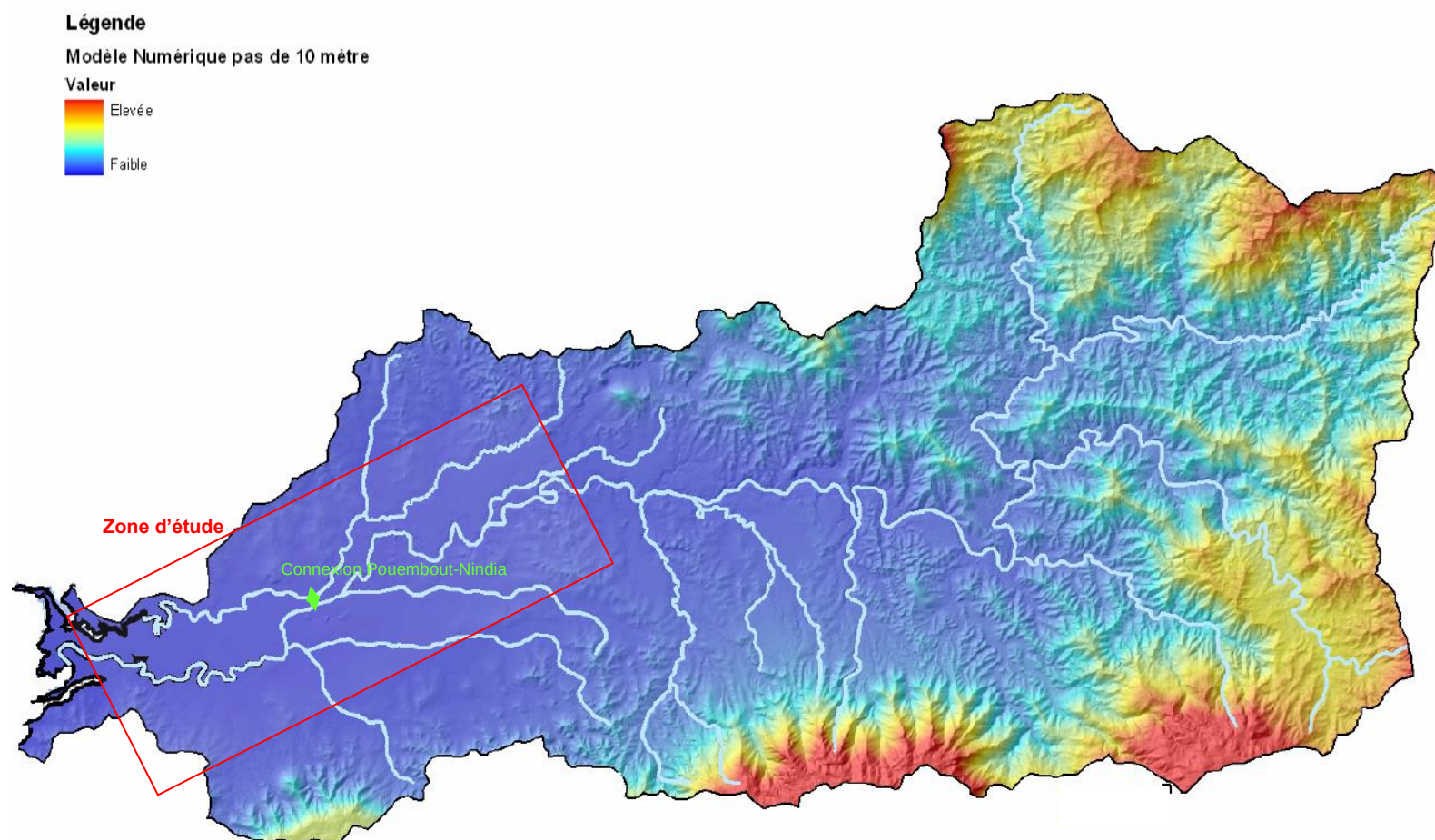
Figure 14 : Bassin versant global de la rivière Pouembout
