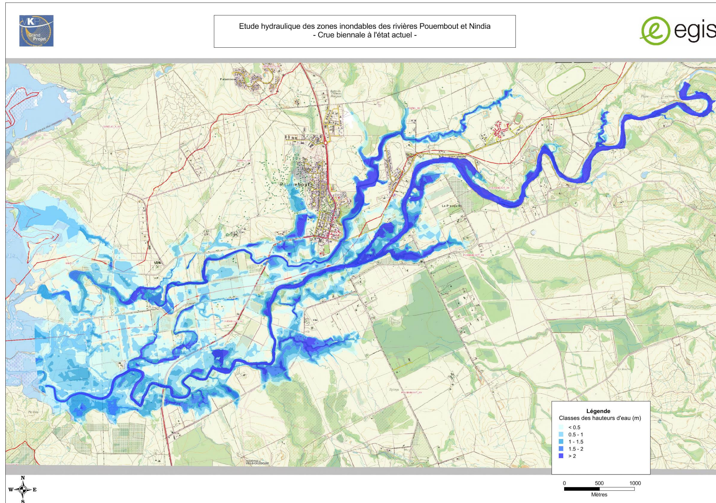
Figure 28 : Cartographie des zones inondables avec iso-hauteurs pour la crue d'ordre de retour Q2 / SactQ2-1
