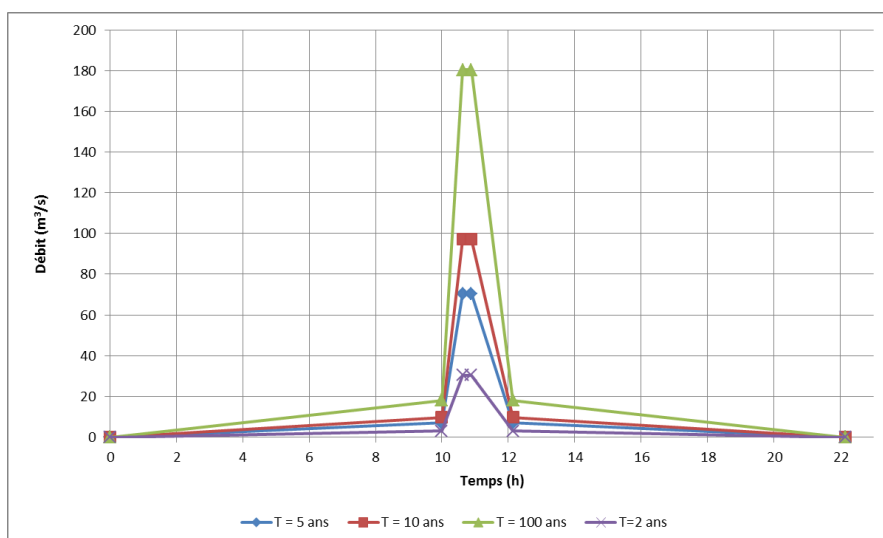
Figure 19 : Description schématique de l'hydrogramme reconstitué : de l'affluent 2 de la rivière Nindia
