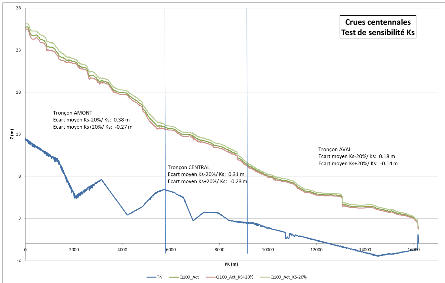
Figure 26 : Profil en long du lit mineur de la Pouembout avec test de sensibilité des coefficients de rugosité
