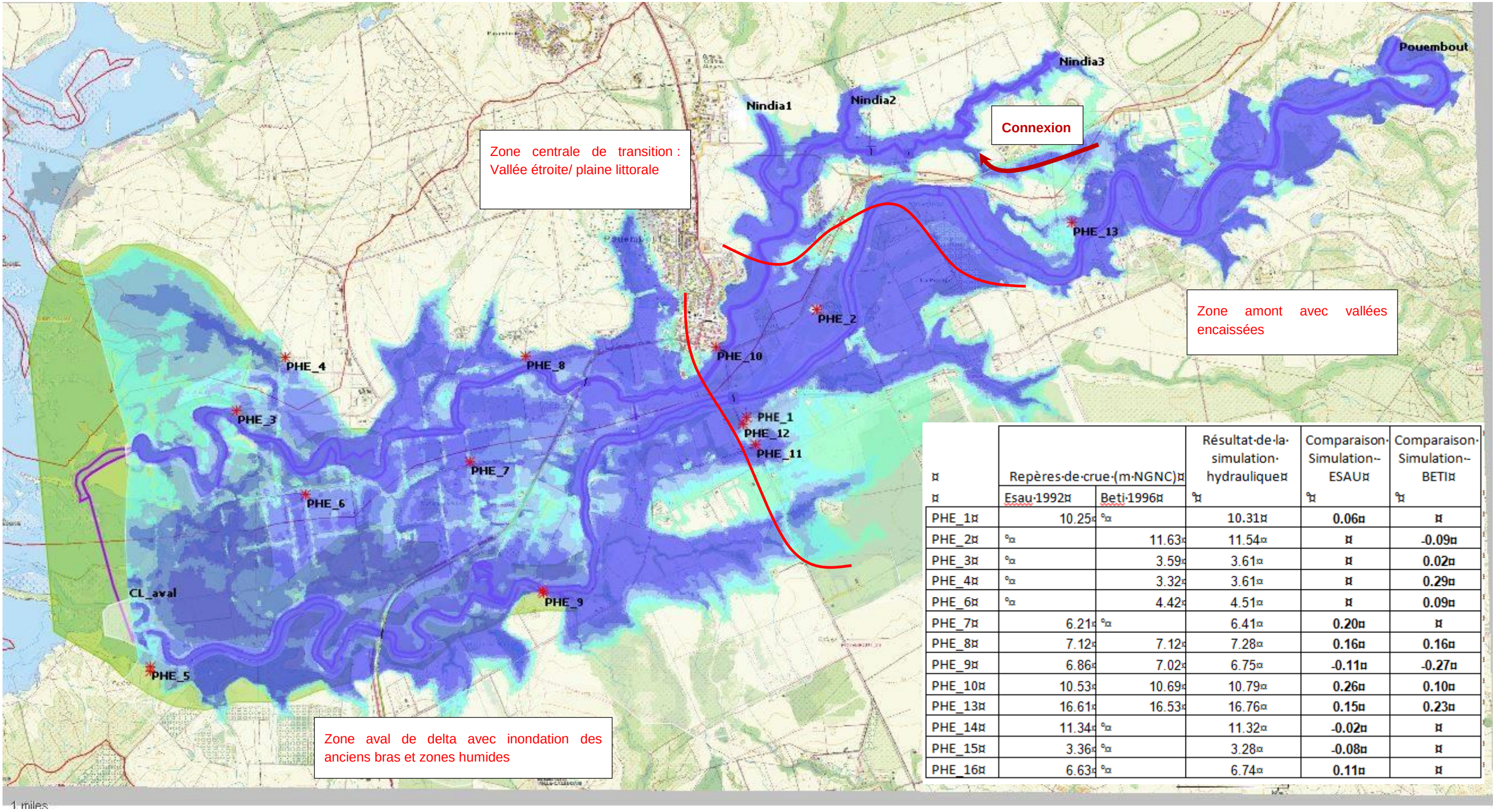
Figure 23 : Résultat de la modélisation pour la crue de calage Cyclones ESAU-BETI
