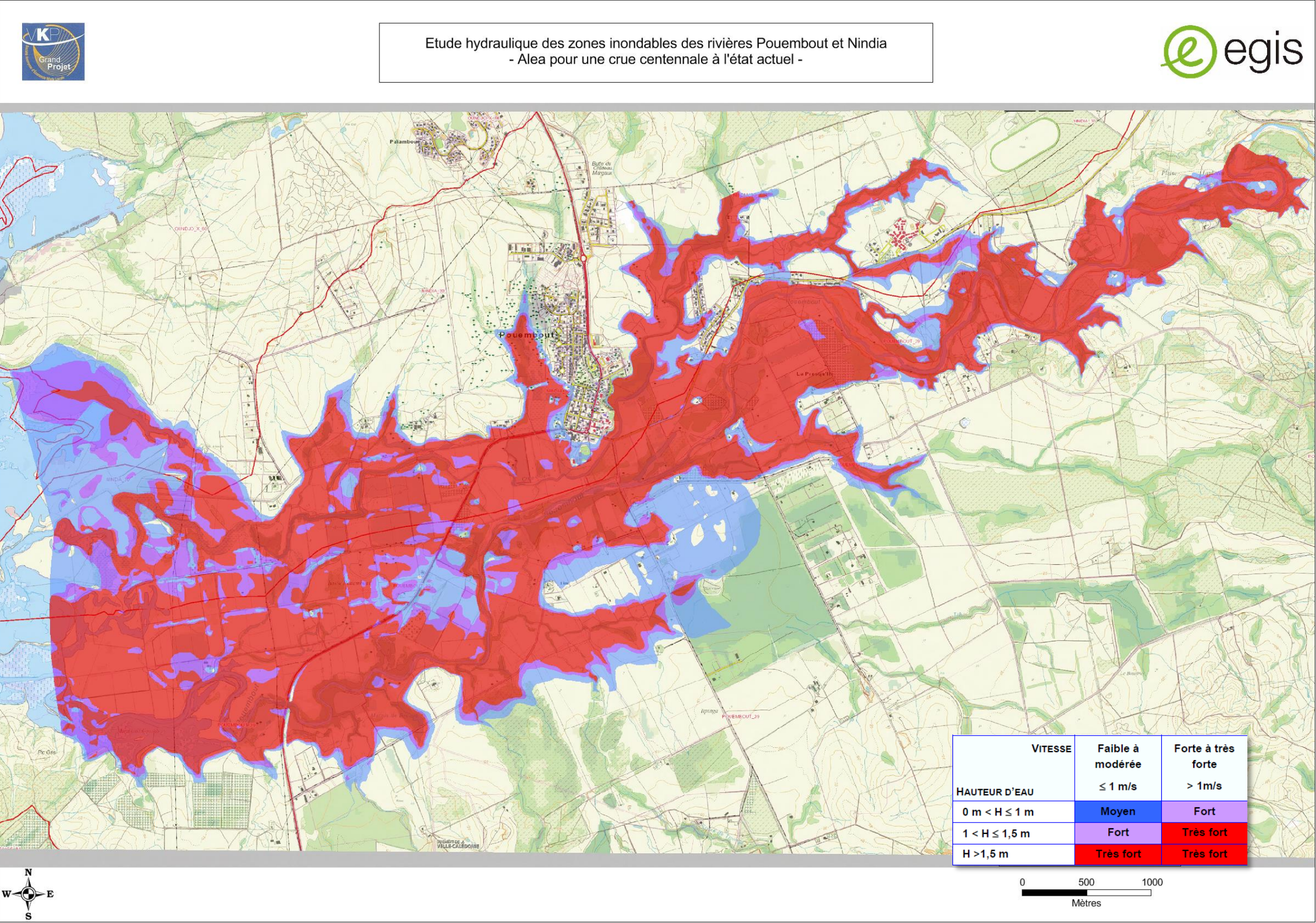
Figure 34 : Cartographie de l'aléa inondation
