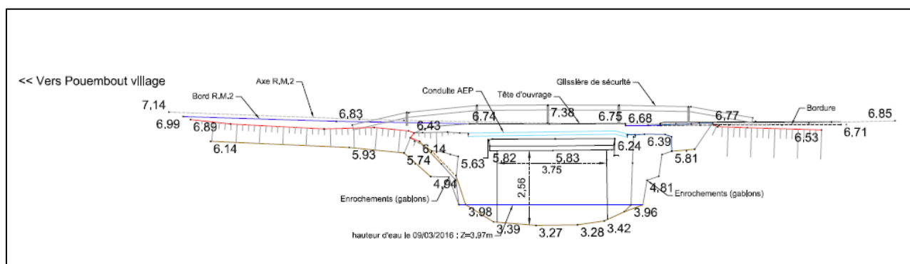
Figure 22 : Exemple ouverture hydraulique du pont OH2 sur la Nindia
