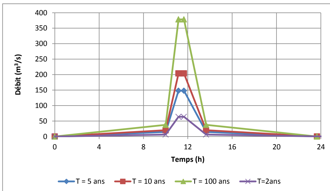
Figure 17 : Description schématique de l'hydrogramme reconstitué de la rivière Nindia
