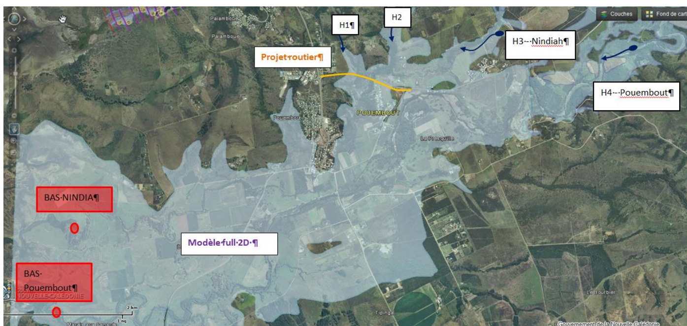
Figure 13 : Injections des hydrogrammes dans le modèle hydraulique
