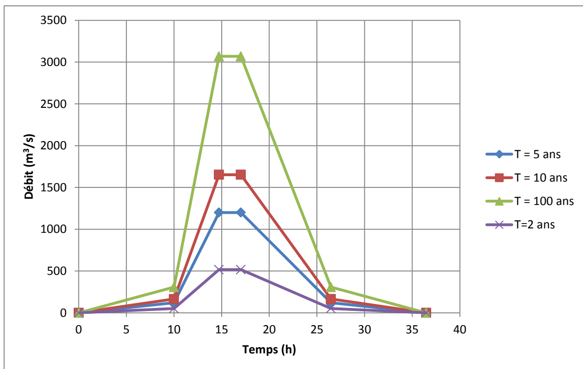
Figure 20 : Description schématique des hydrogrammes reconstitués: de la rivière Pouembout
