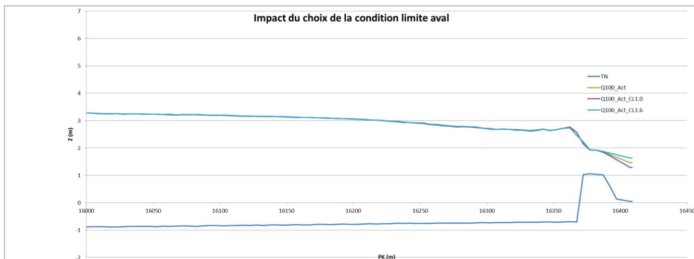
Figure 25 : Profil en long sensibilité de la condition limite aval
