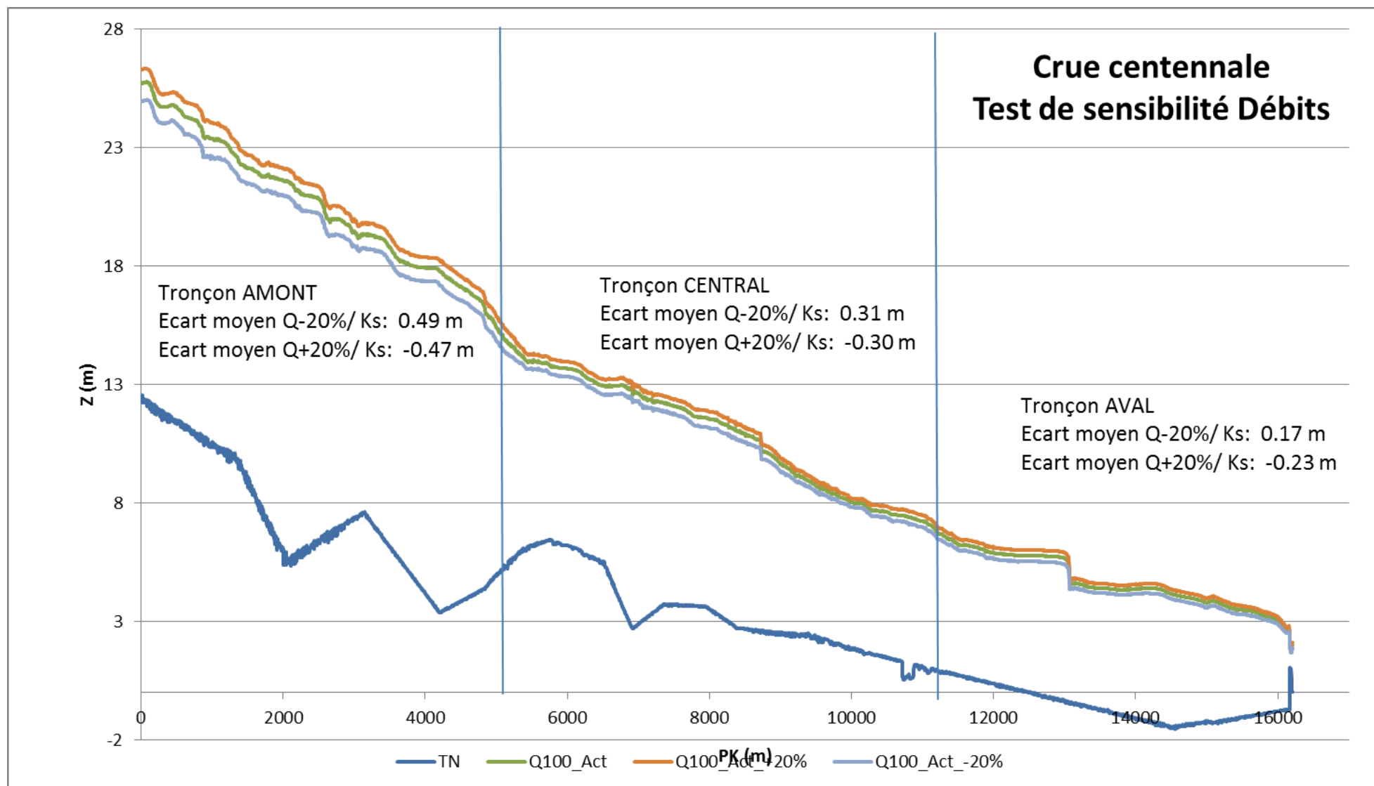
Figure 27 : Profil en long du lit mineur de la Pouembout avec test de sensibilité débits injectés
