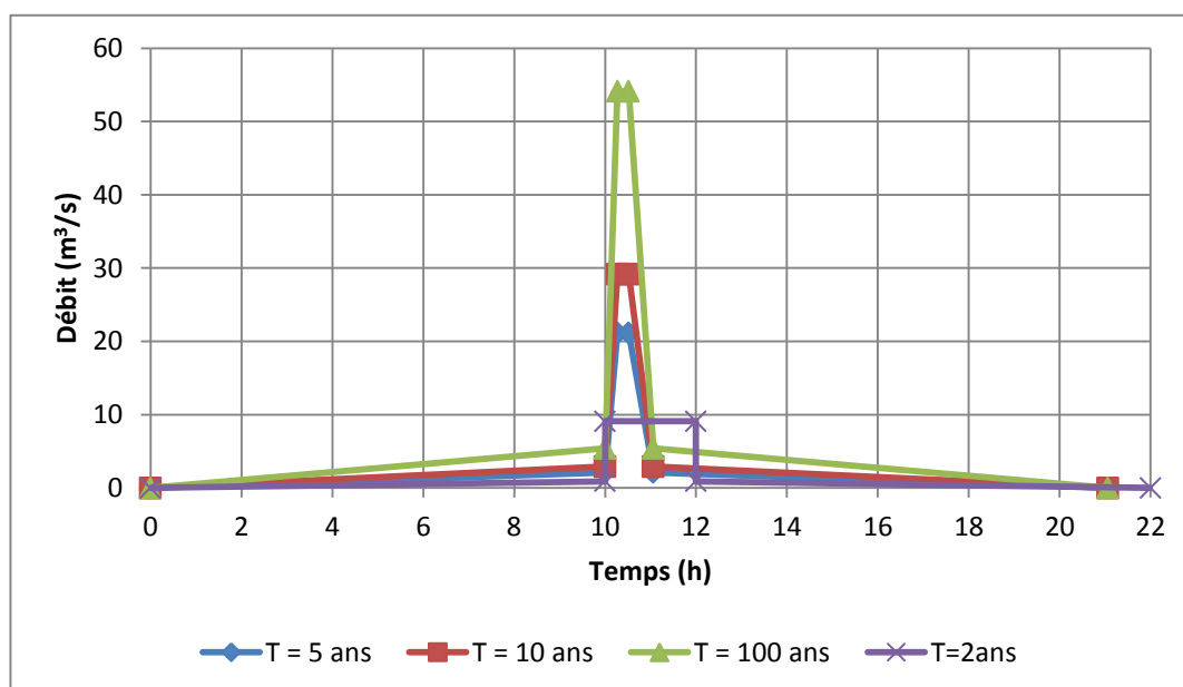
Figure 18 : Description schématique de l'hydrogramme reconstitué : de l'affluent 1 de la rivière Nindia
