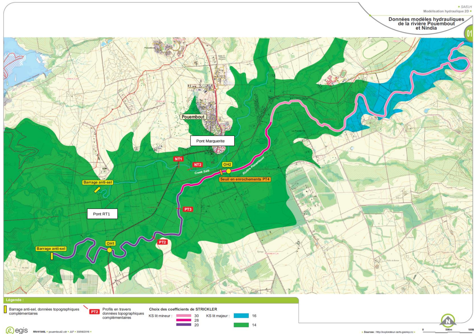
Figure 4 : Principaux ouvrages et coefficients de Strickler dans le lit mineur et majeur
