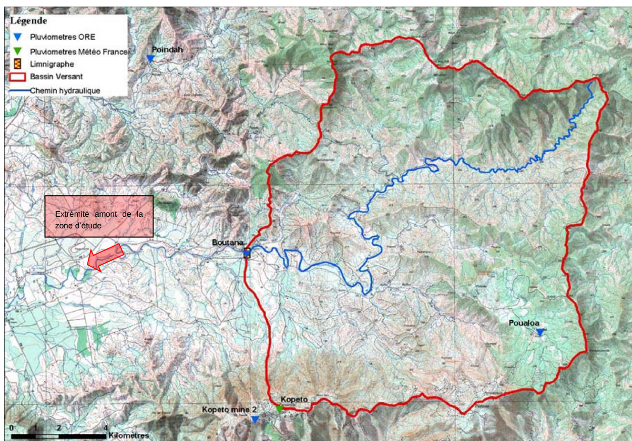
Figure 15 : Localisation du bassin versant de la station de BOUTANA (13)
