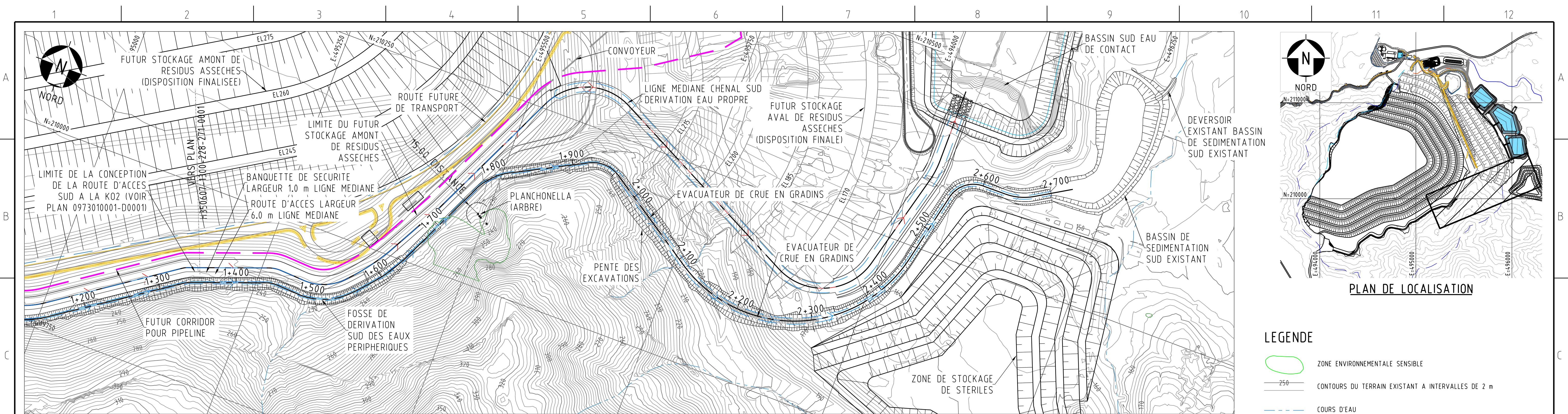
PLAN - FOSSE DE DERIVATION SUD DES EAUX PERIPHERIQUES ECHELLE 1/2500
