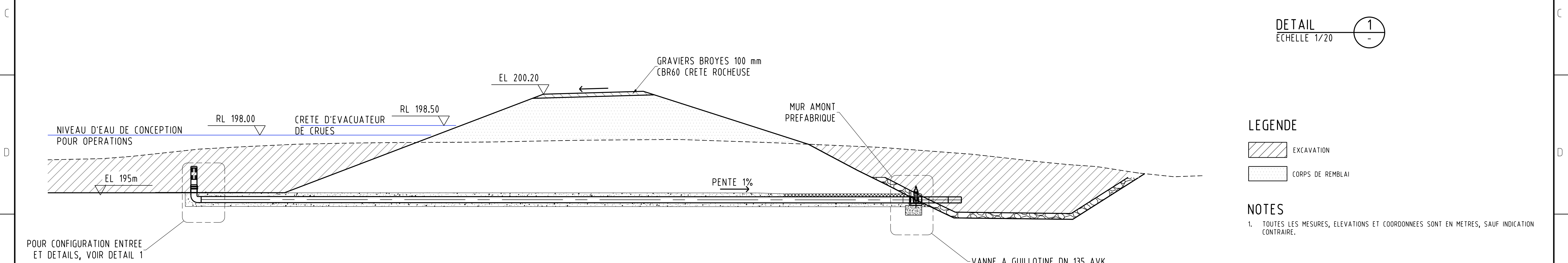
SORTIE TUYAU DECANTATION
