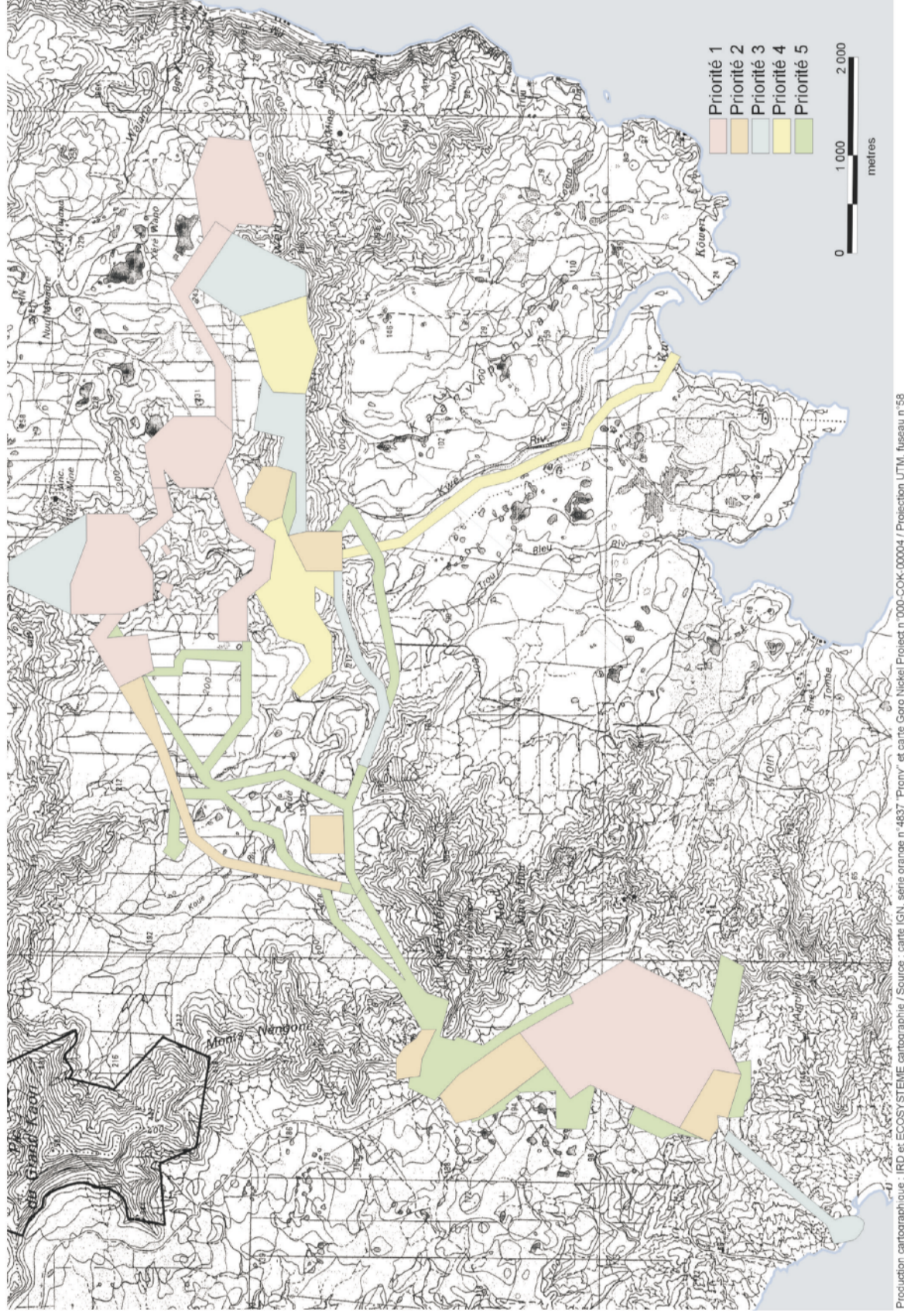
fig. 1 : Plan des zones d'étude du site de Goro Nickel
