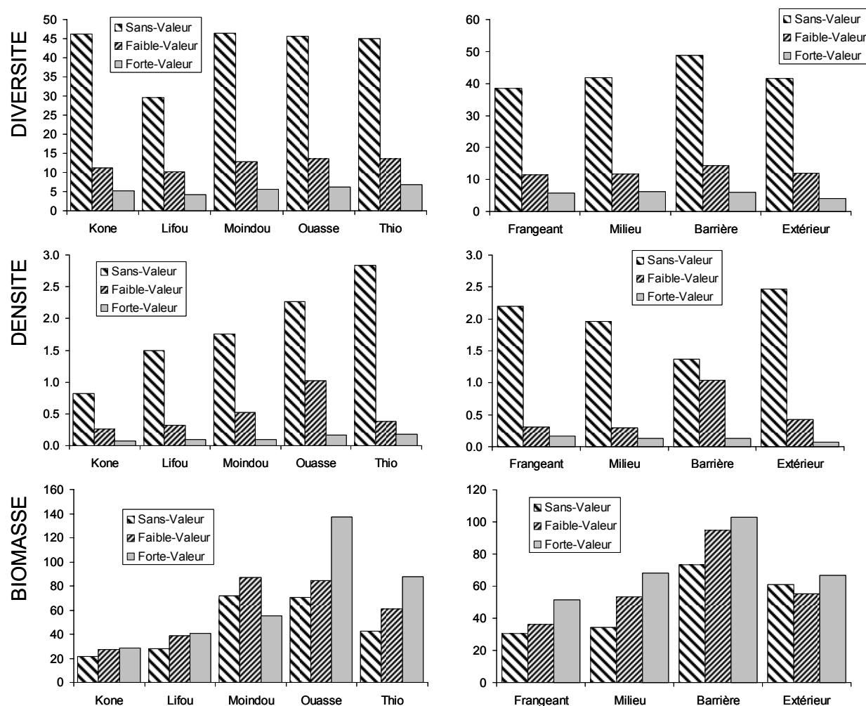
Figure 16 : distribution des espèces en fonction de leur valeur commerciale suivant les sites et les types de récif. Basé sur les données IRD. Diversité en nombre d'espèces / transect ; Densité en poissons / m² ; Biomasse en g/m²
