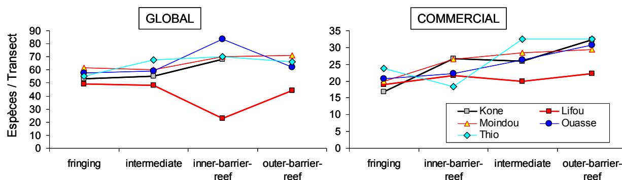
Figure 8 : richesse spécifique (nombre d'espèces / transect) en fonction du site et du type de récif. « Global » comptages de toutes les espèces (IRD) ; « Commercial » comptages restreint (CPS)
