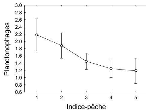
Figure 19 : effet de la pêche sur la biomasse (échelle log) des planctonophages. L'indice 1 indique le niveau de pêche le plus faible et 5 le plus fort.
