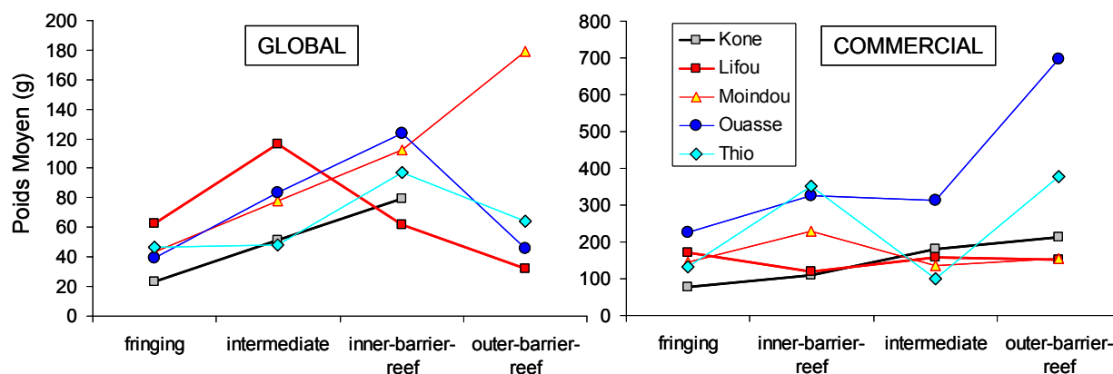
Figure 11 : poids moyen des poissons (g) en fonction du site et du type de récif. « Global » : comptages de toutes les espèces (IRD) ; « Commercial » : comptages restreints (CPS)
