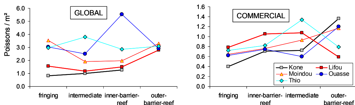
Figure 9 : densité (poissons / m 2 ) en fonction du site et du type de récif. « Global » : comptages de toutes les espèces (IRD) ; « Commercial » : comptages restreints (CPS)
