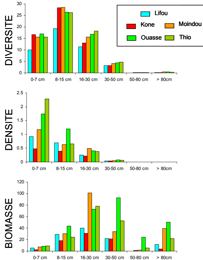
Figure 14 : distribution des catégories de taille en fonction du site, données IRD seulement. Diversité en nombre d'espèces / transect ; Densité en poissons /m² ; Biomasse en g/m²
