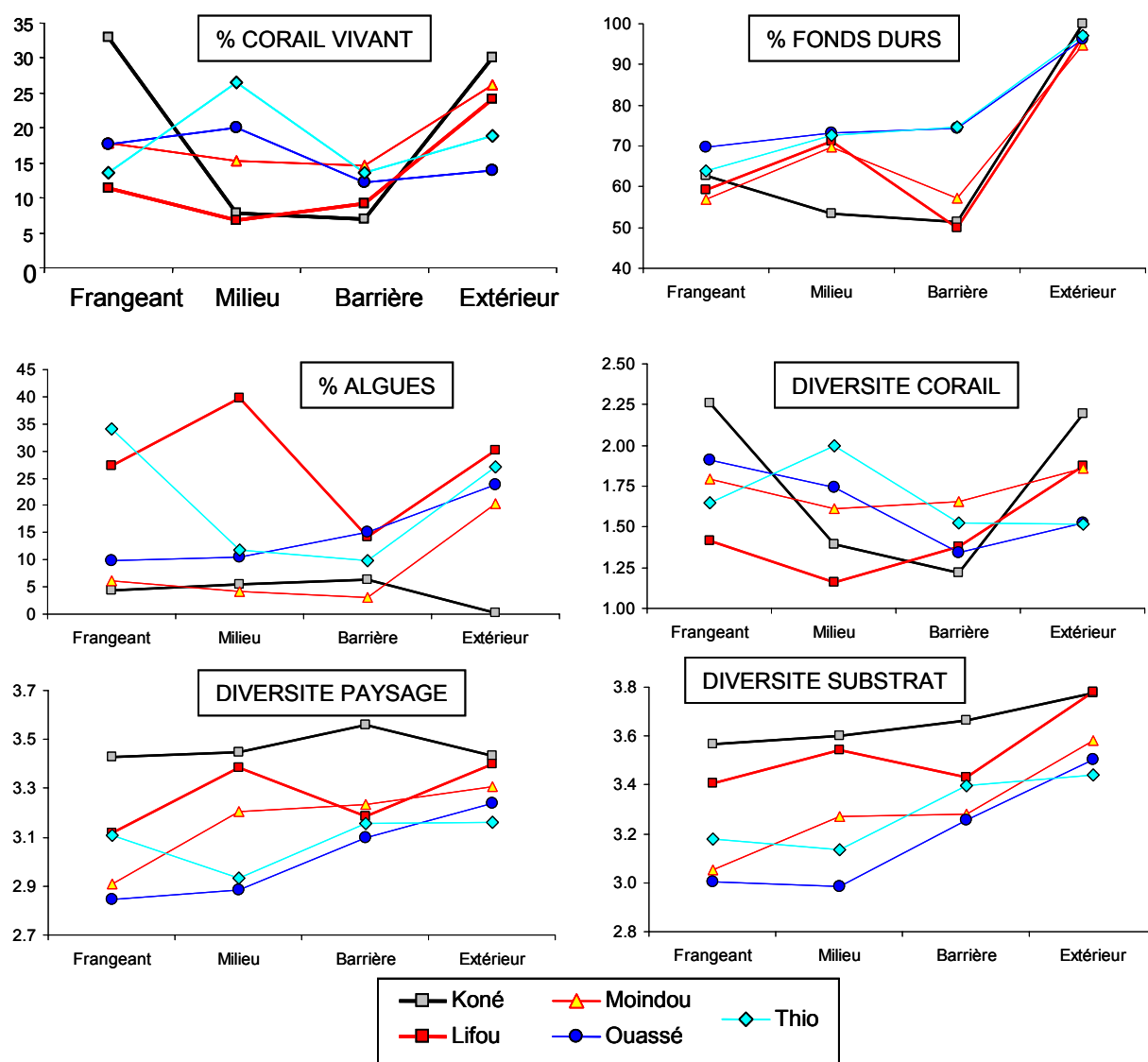
Figure 18 : principales caractéristiques de l'environnement sur les stations. Les ordonnées sont des % de recouvrement pour « % Corail », « % Fonds durs », « % Algues » et sont la valeur de l'indice de Shannon pour les diversités
