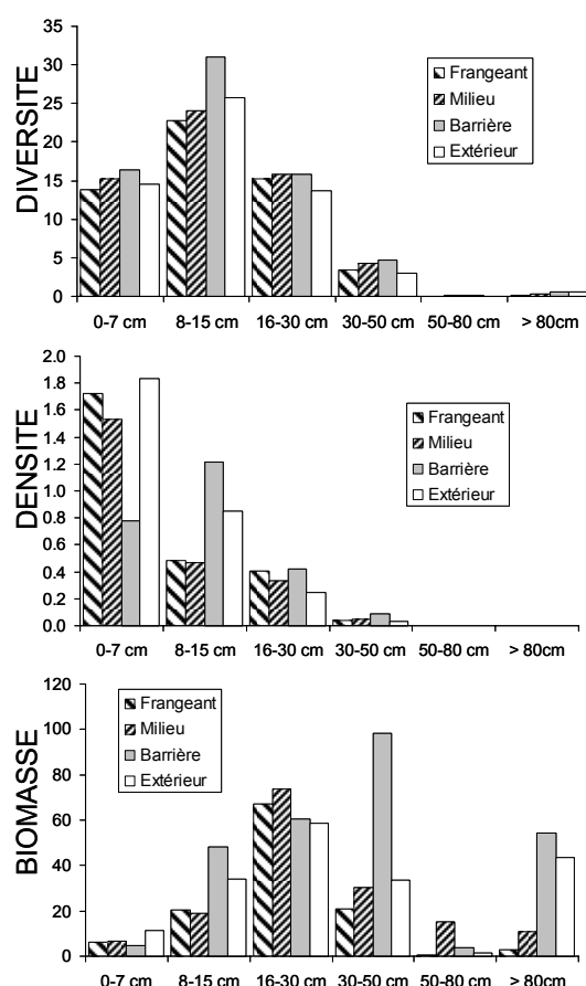
Figure 15 : distribution des catégories de taille en fonction du type de récif, données IRD seulement. Diversité en nombre d'espèces / transect ; Densité en poissons /m 2 ; Biomasse en g/m 2
