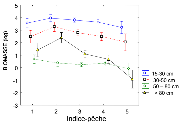
Figure 19 : effet de la pêche sur la biomasse (échelle log) des poissons en fonction de la taille de l'espèce. L'indice 1 indique le niveau de pêche le plus faible et 5 le plus fort.
