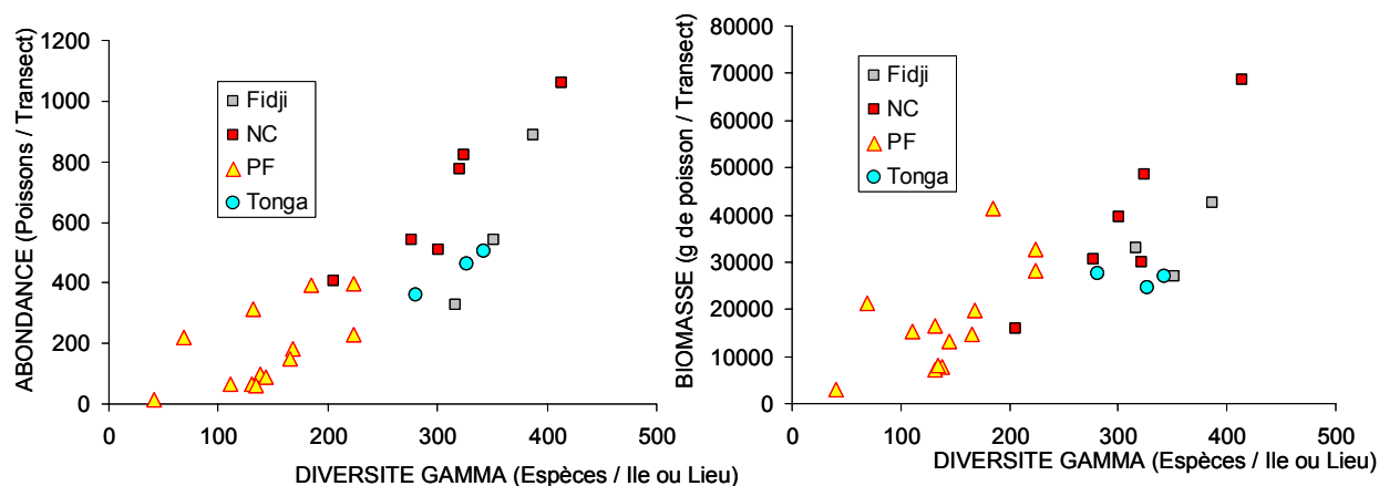
Figure 23 : relations entre densité (abondance), biomasse et diversité à grande échelle. Chaque point représente un site d'étude (chaque site comprend un grand nombre de stations). La diversité gamma représente l'ensemble des espèces échantillonnées sur le site.
