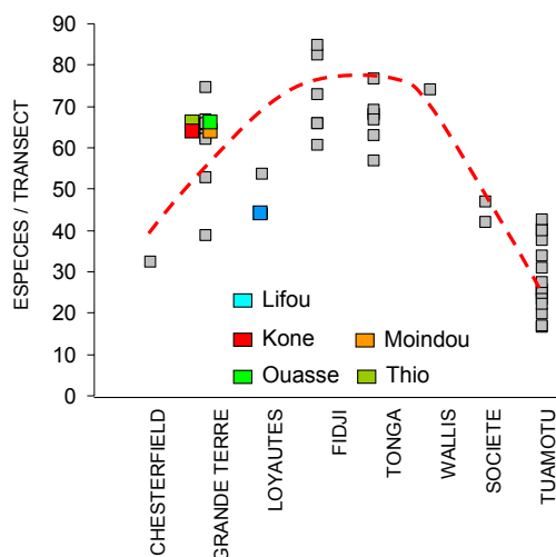
Figure 21 : comparaison des valeurs moyennes de diversité obtenues lors de la présente étude avec d'autres sites du Pacifique Sud. Les sites sont rangés d'ouest en est.
