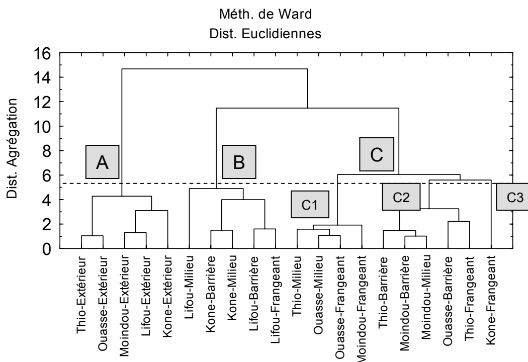
Figure 17 : classification des stations en fonction des principales caractéristiques de l'environnement (Tableau 9)
