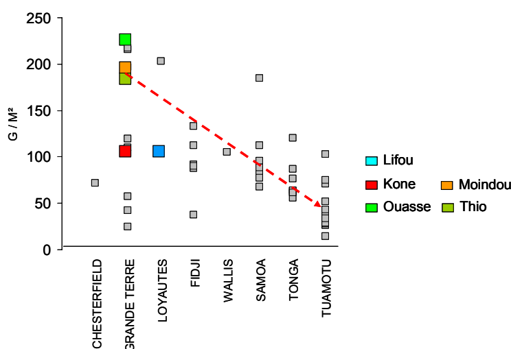
Figure 24 : comparaison des valeurs moyennes de biomasse obtenues lors de la présente étude avec d'autres sites du Pacifique Sud. Les sites sont rangés d'ouest en est.
