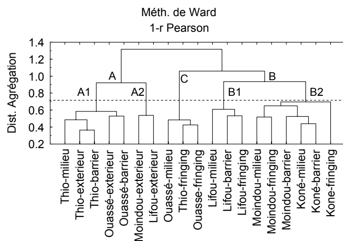
Figure 7 : Classification des zones en fonction de la composition spécifique (présence / absence). Agrégation par la méthode de Ward, distance « r de Pearson ».
