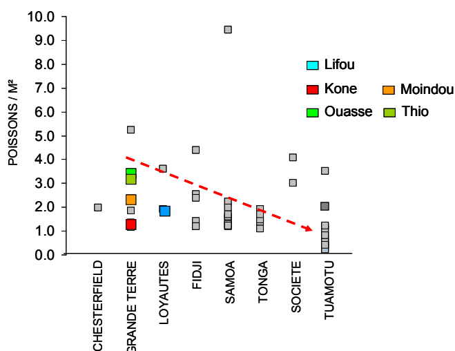
Figure 22 : comparaison des valeurs moyennes de densité obtenues lors de la présente étude avec d'autres sites du Pacifique Sud. Les sites sont rangés d'ouest en est.
