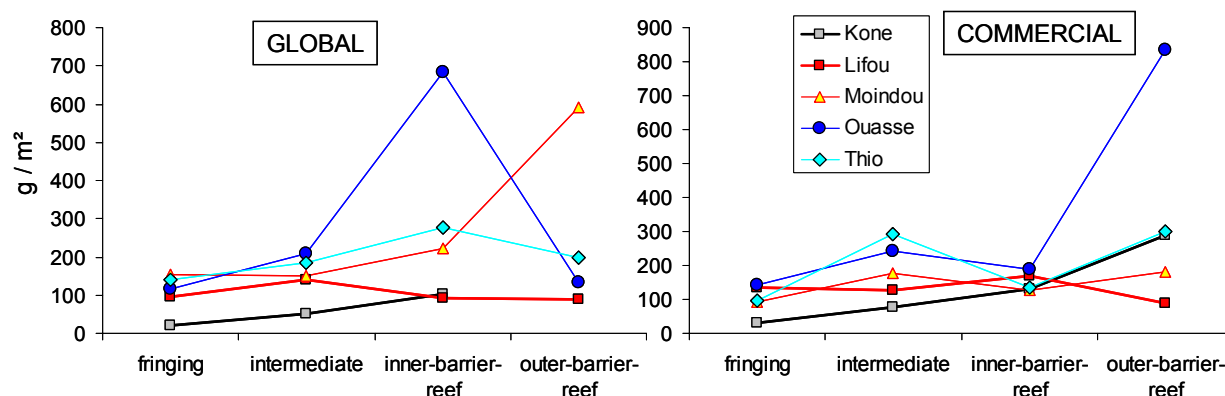
Figure 10 : biomasse ( \text{g} / \text{m}^2 ) en fonction du site et du type de récif. « Global » : comptages de toutes les espèces (IRD) ; « Commercial » : comptages restreints (CPS)
