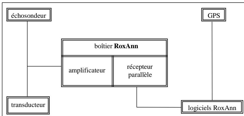
Figure 2 : Principaux éléments du système RoxAnn.
