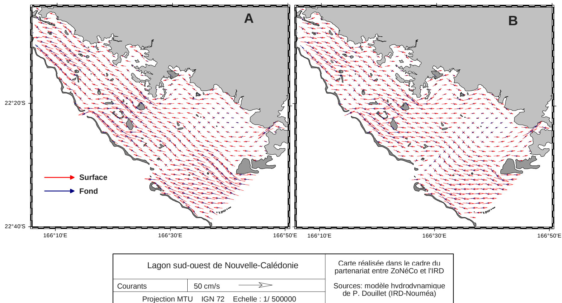
Figure I-10 Courants générés en surface et au fond sur le SLNC par un vent de 8m.s-1. A vent de direction typique Alizé (110° N), B vent d'Ouest (270° N). Données issues du modèle MARS3D implanté sur le SLNC
