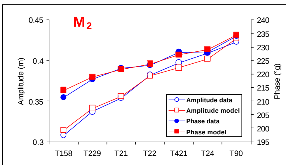
Figure 4 : Comparaison des amplitudes et phases de l'onde M_2
