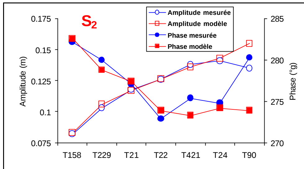
Figure 5 : Comparaison des amplitudes et phases de l'onde S_2
