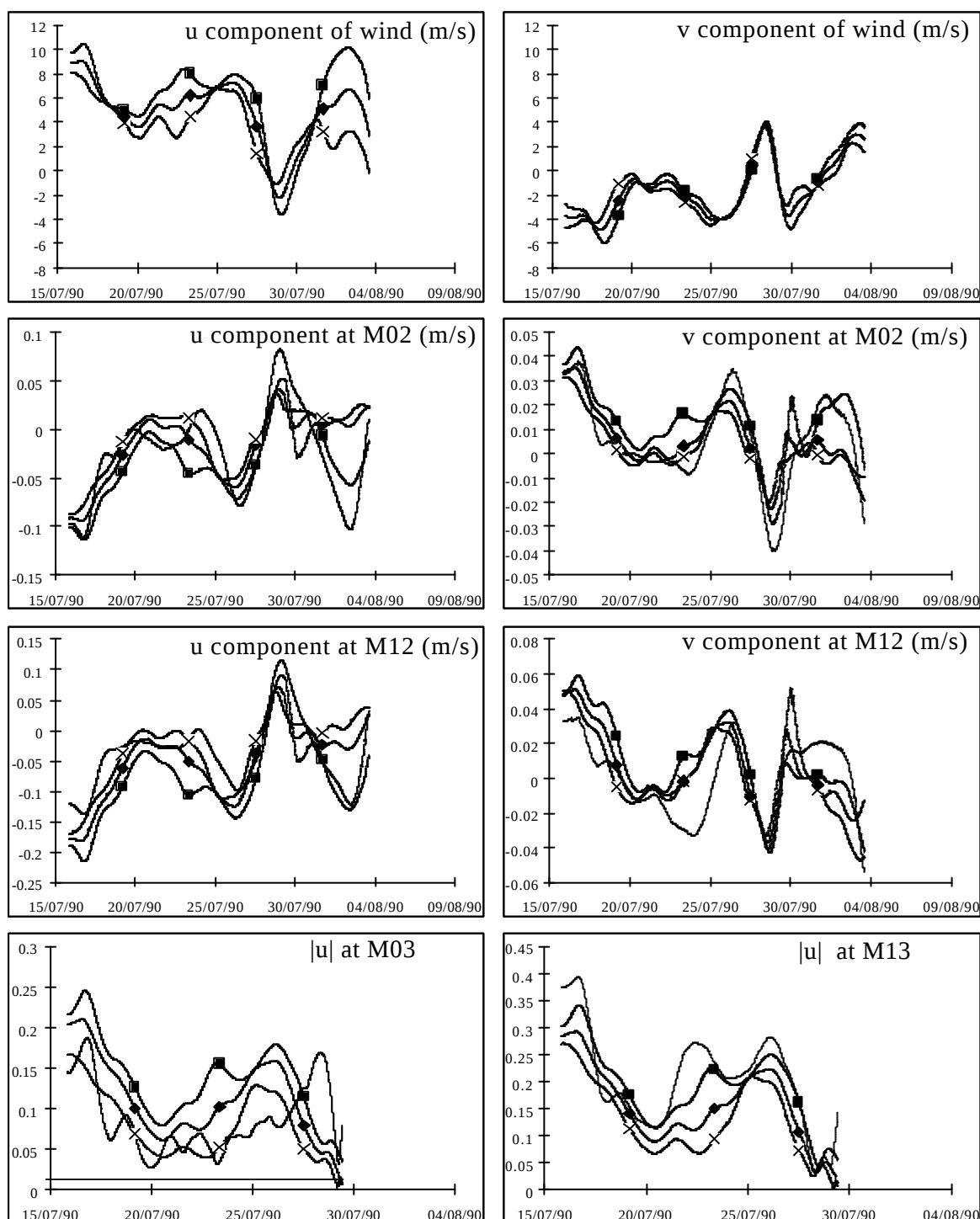
Figure 6 : Comparaison entre les courants mesurés et calculés pour 3 vents différents, ■ W30, ◆ W31, ✕ moyenne de W30 et W31.
