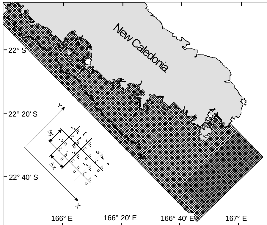
Figure 2 : Domaine de simulation. Schéma de la grille Arakawa C modifiée.
