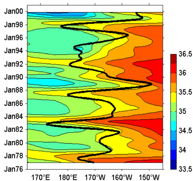
Figure 2. Evolution de la salinité de surface de la mer de 1976 à 2000 à 17°S. La ligne continue représente les variations de la SOI, indicatrices des événements El Niño et La Niña.
