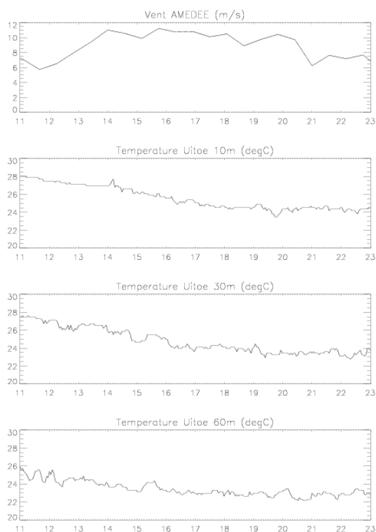
Figure 6: Etude de l'épisode d'upwelling de février 2002, le plus marqué depuis l'installation des capteurs thermiques de profondeur à Uitoé. La profondeur d'origine des remontées d'eau est estimée à 80 m et la vitesse de remontée de l'ordre de 1 à 2 mètres par heure.
