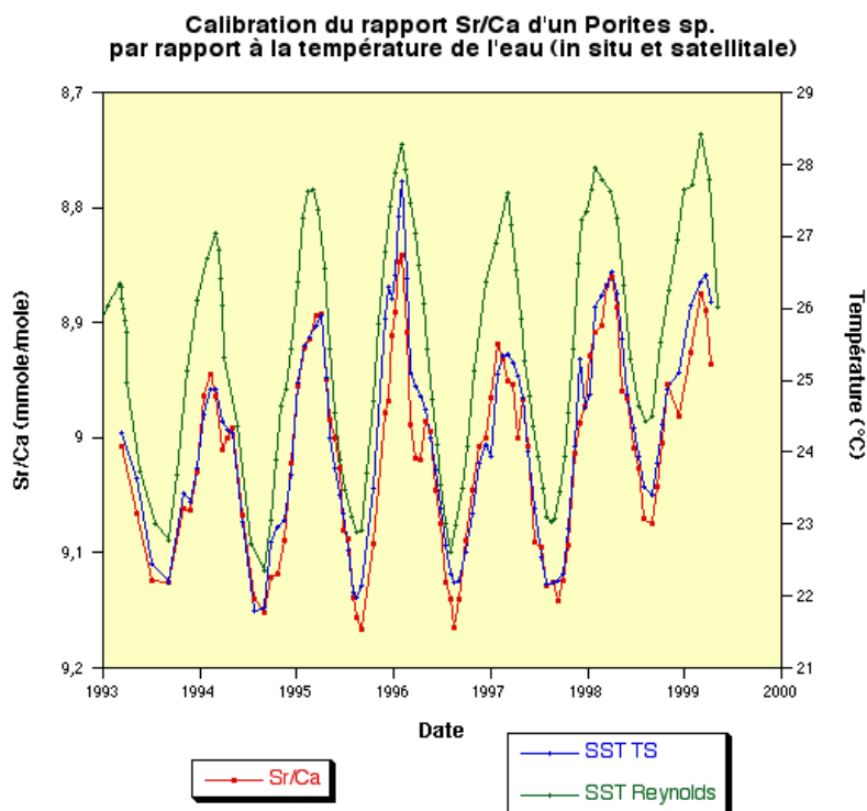
Figure 7. Cette figure montre l'excellente relation qui existe entre les mesures chimiques (le rapport Sr/Ca en rouge) et la série temporelle de température de la mer relevée au Phare Amédée (courbe bleue). L'utilisation de mesures plus globales tel que le produit de température de Reynolds (courbe verte) ne permet pas une aussi bonne reconstitution de la température océanique à partir des mesures corallienne.
