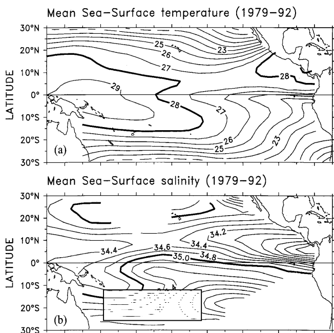
Figure 1. Température et salinité de surface. Le rectangle indique la zone d'étude.
