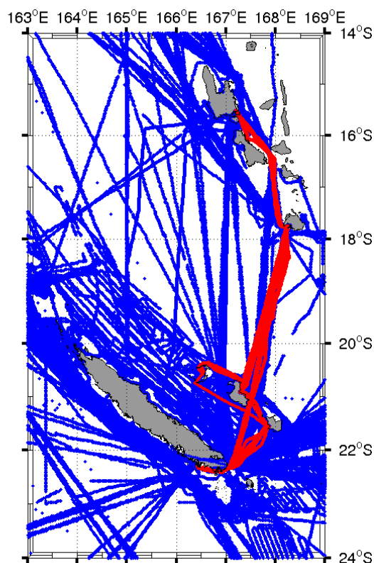
Figure 5: Position des mesures de température et de salinité de surface de la mer effectuées au cours de l'année 2003 grâce aux thermosalinographes installés sur les navires marchands. Les points en rouge représentent les mesures faites à partir du Havannah. Les points en bleu représentent les mesures effectuées par l'ensemble des bateaux gérés par l'IRD.
